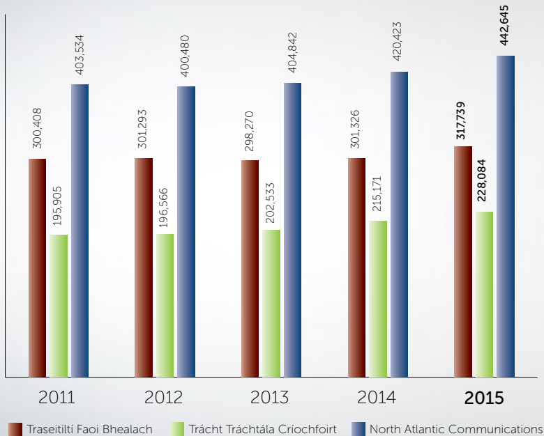
Gníomhaíocht Aerthráchta
