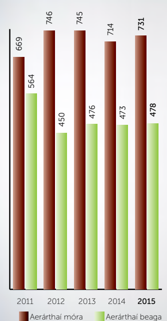
Aerárthaí Cláraithe
