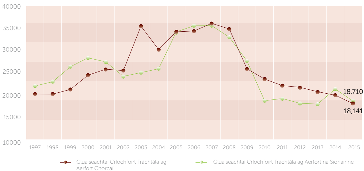
Gluaiseachtaí Críochfoirt Tráchtála ag Aerfort na Sionainne agus ag Aerfort Chorcaí (1997 go 2015)
