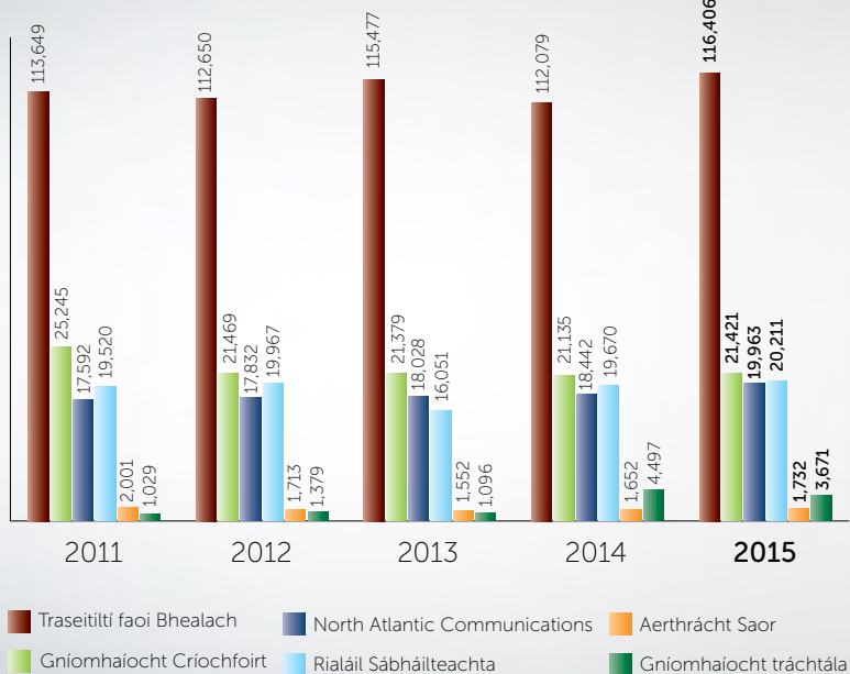
Láimhdeachas €'000
